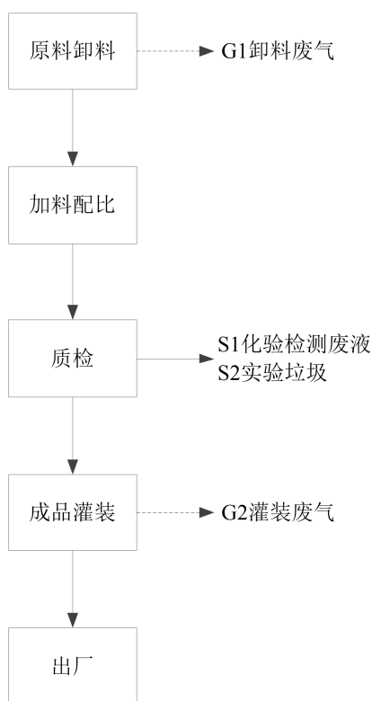
图 2-4 制冷剂工艺流程图
