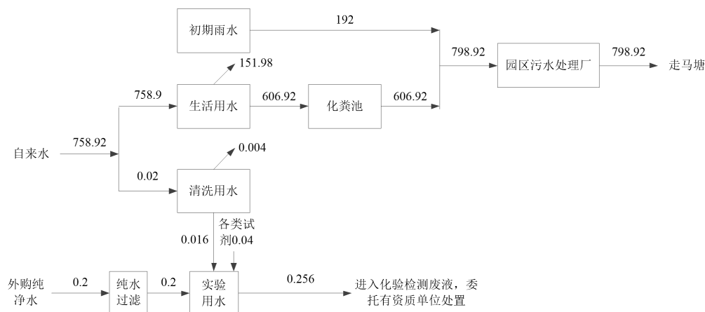
图 2-3 本项目建成后全厂水平衡图 (m 3 /a)
