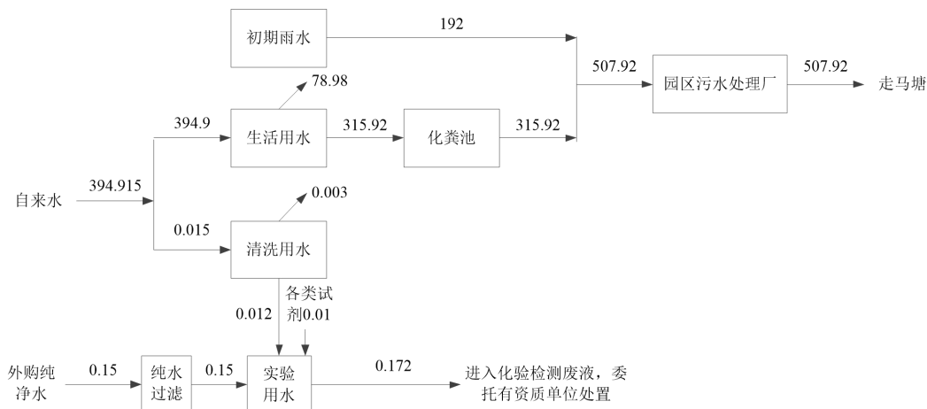
图 2-2 本项目水平衡图 (m 3 /a)
