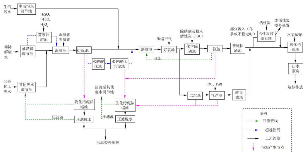
图 4-1 污水处理厂废水处理工艺流程图
